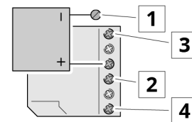
Pinbelegung bei Finder 26.01.8.024 mit DC-Adapter 026.9.024
