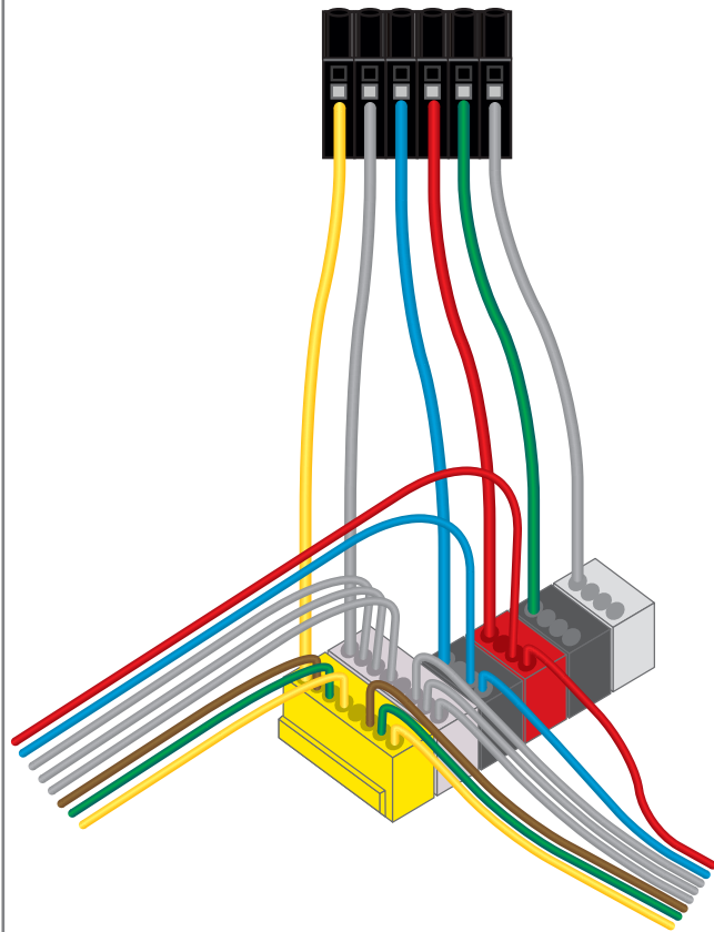
Detailzeichnung Anschluss BM-ZK
