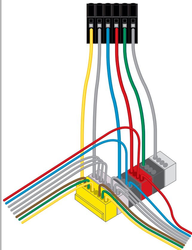
Detailzeichnung Anschluss BM-Z
